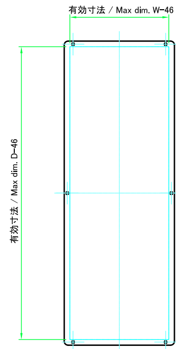
パネル表面 / Panel Frontside
